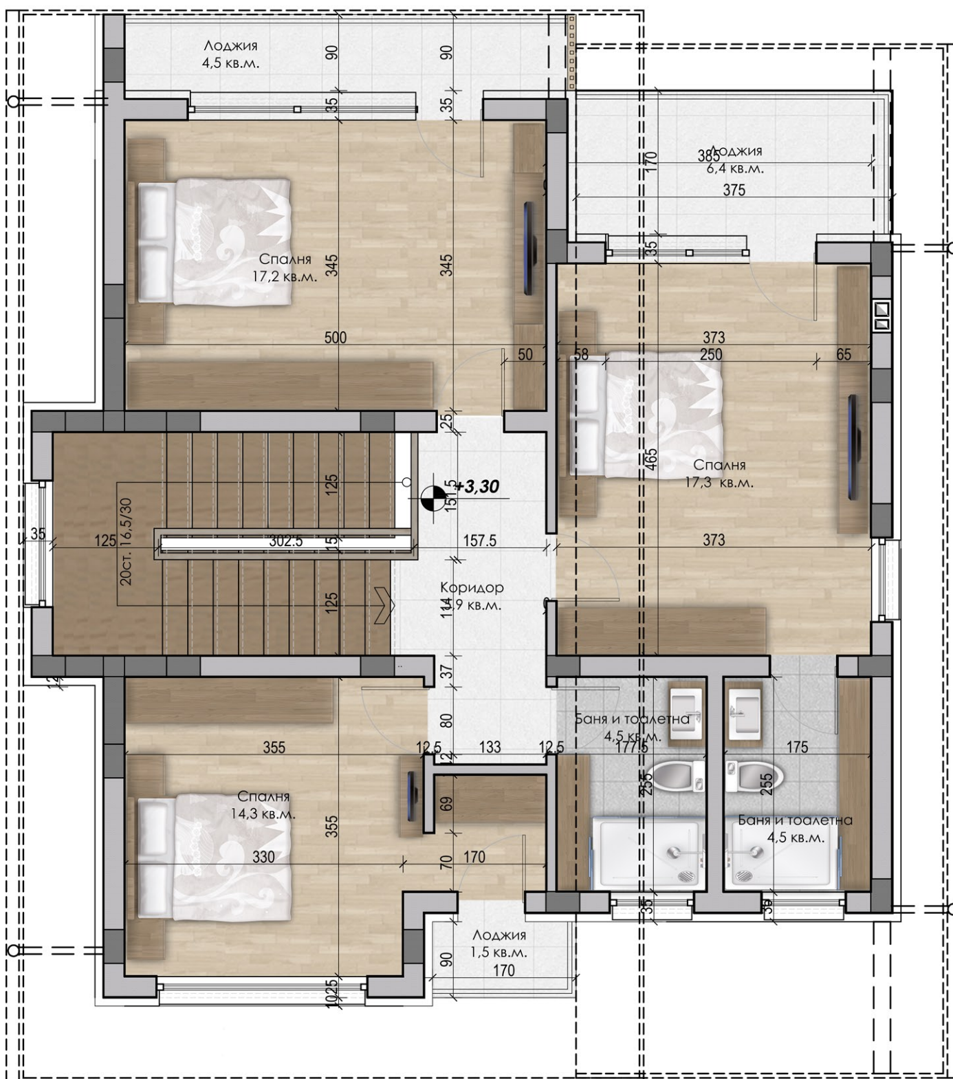
ЕДНОФАМИЛНА КЪЩА РАЗПРЕДЕЛЕНИЕ +3,30
